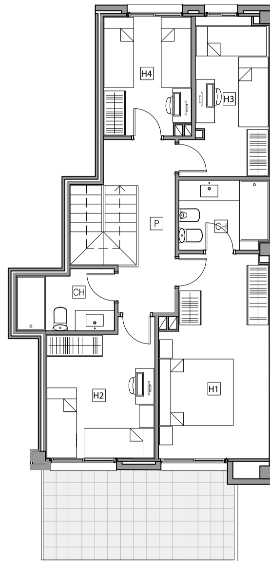
▲ Planta primera
