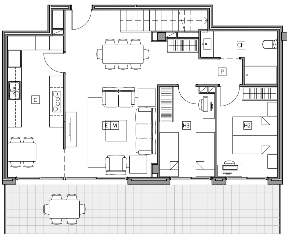
▲ Planta segunda
